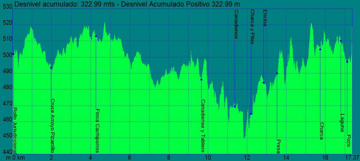
Perfil del paseo por camino Hocinillo, Vereda Cuerda de Berenga y camino de Aldeacentenera
